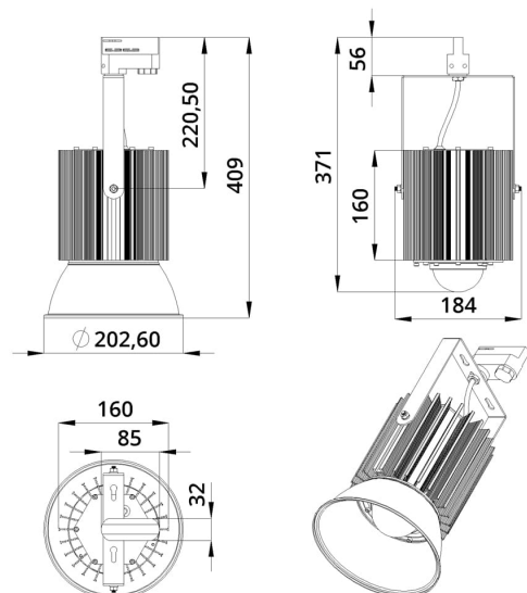
Габаритный чертёж
