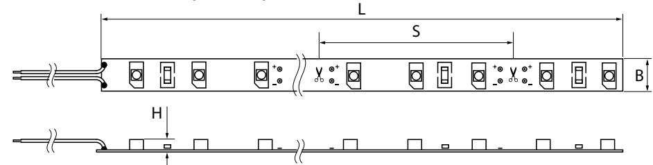
Рис. 1 Лента светодиодная
